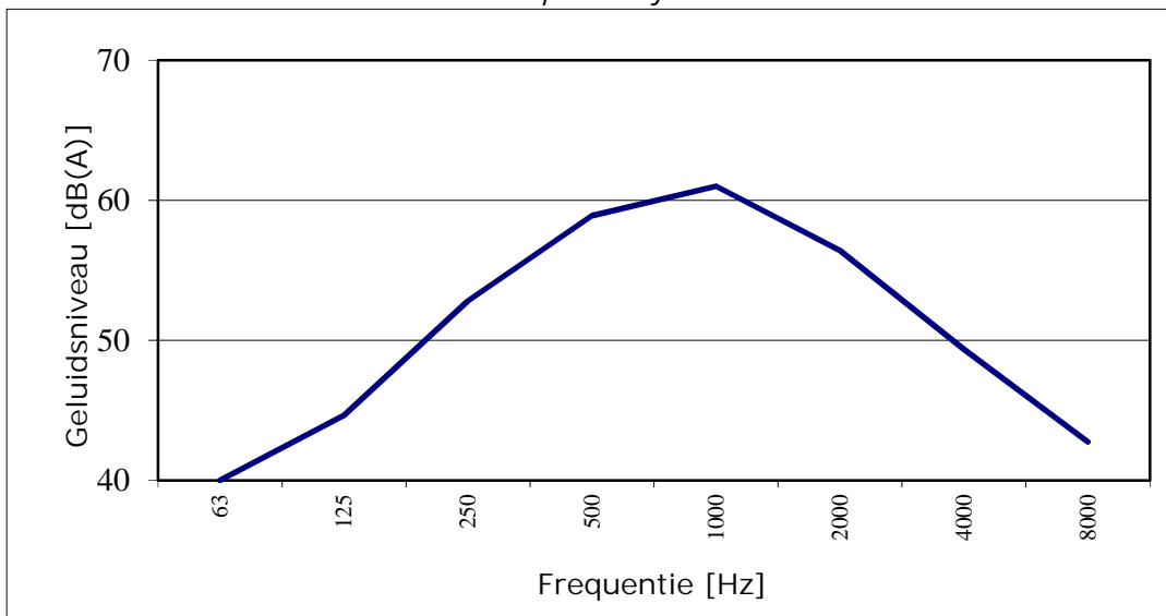
Octaafbandspectra bij 44 km/uur
