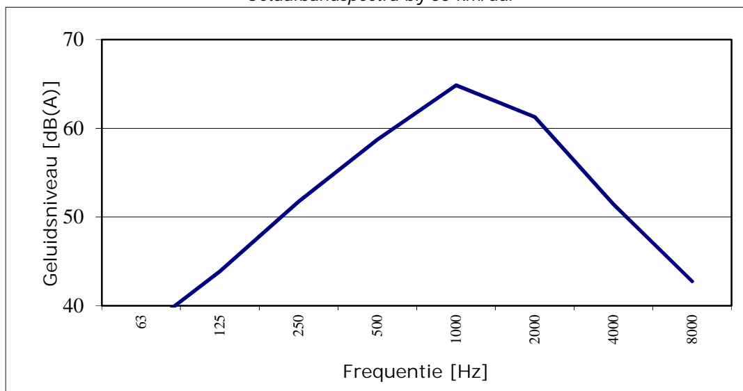
Octaafbandspectra bij 55 km/uur
