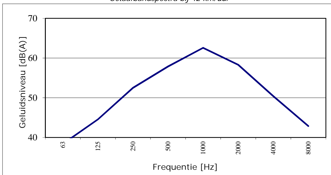
Octaafbandspectra bij 42 km/uur
