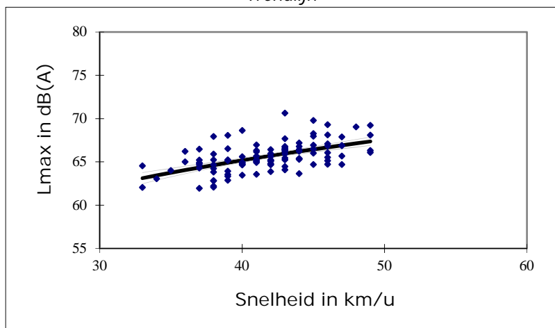
Trendlijn
